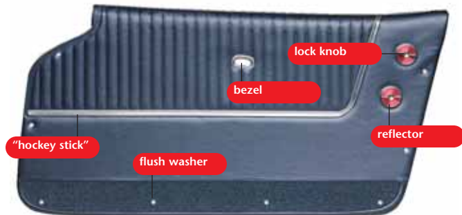
63-64 Deluxe Door Panel
