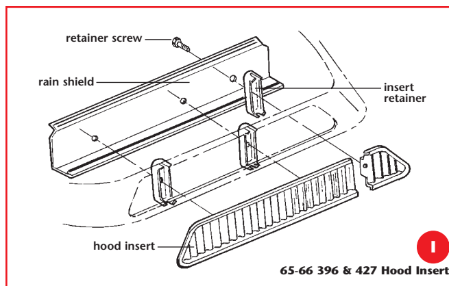
65-66 396 & 427 Hood Insert
